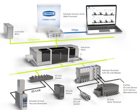
Интеграция Schmalz Connect Suite в архитектуру системы
